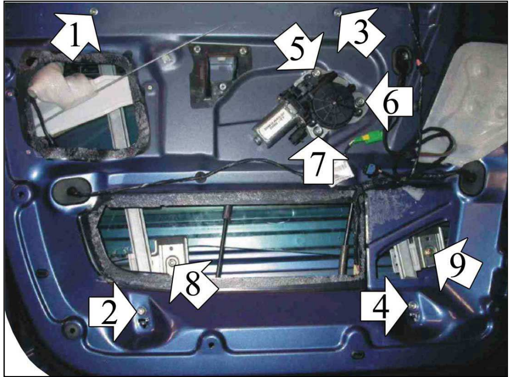
left door - portière gauche - linke tür - puerta lado izquierdo - porta esquerda - porta lato sinistro
